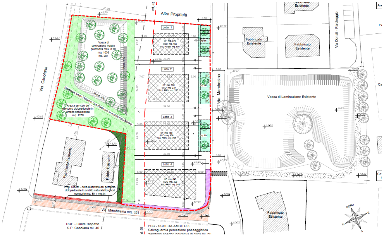
Figura 3: Planimetria dell'intervento
